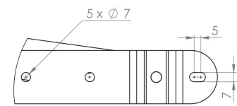
SZCZEGÓŁ A SKALA 1 : 2
