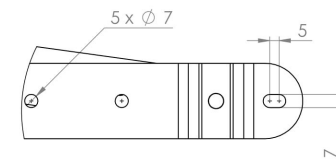
SZCZEGÓŁ A SKALA 1:2
